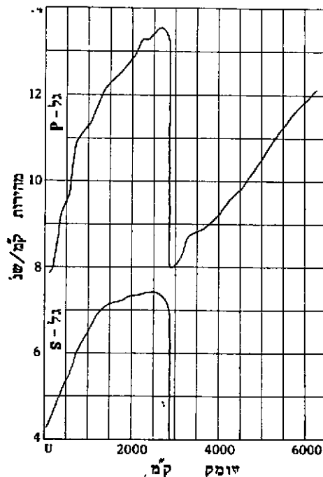
גלים סיכטיים ג' P-γ (= גלים פרימאריים, ראשוניים) — גלים ארכיים; ג' S-γ (= גלים סקונדאריים, שניוניים) — גלים רחביים, שאינם מתפשטים אלא במוצק. שהירות ההתפשטות של שני סוגי הגלים נדלה והולכת עם החדירה לעומק עד לגבול הנרעון
